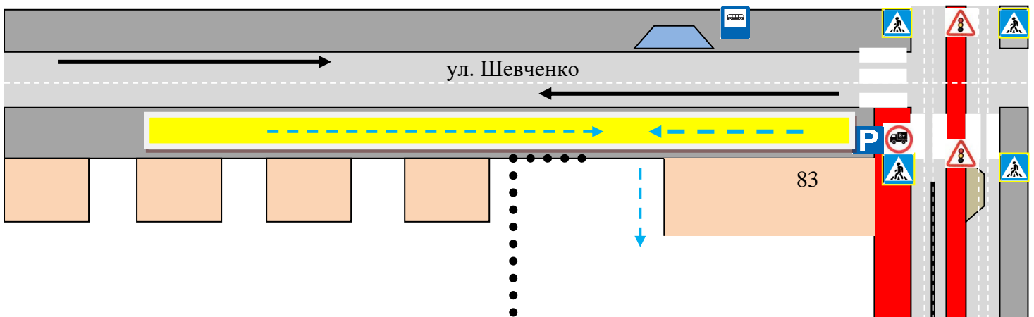
План-схема движения транспортных средств и детей при проведении дорожных ремонтно-строительных работ вблизи образовательной организации.
